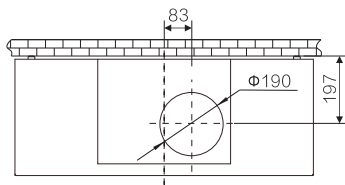
图（3）橱柜及吊顶开孔俯视图
