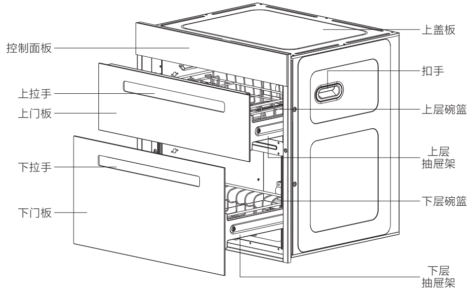
ZTD100-H13结构示意图
