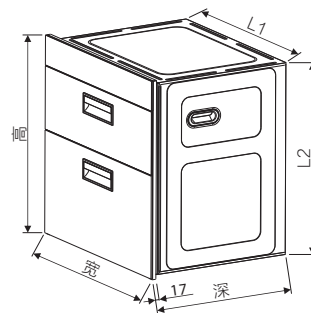
产品尺寸图
