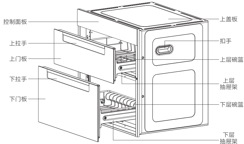
ZTD100-H13结构示意图
